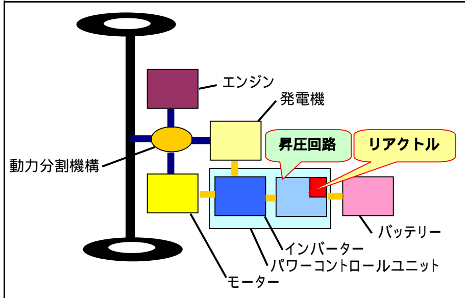
図1. リアクトルの搭載場所
