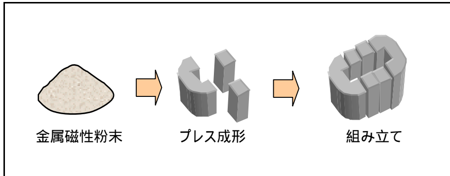
図2. リアクトル用鉄心の製造工程
