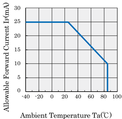
Fig1. I_F / T_a
