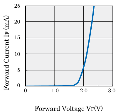
Fig2. I_F / V_F
