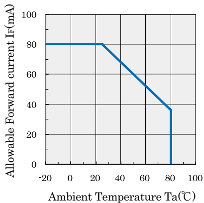
図1. 許容順電流
